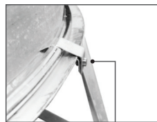
B4: Bắt bulông bát kẹp, giữ thân bồn với chân bồn
